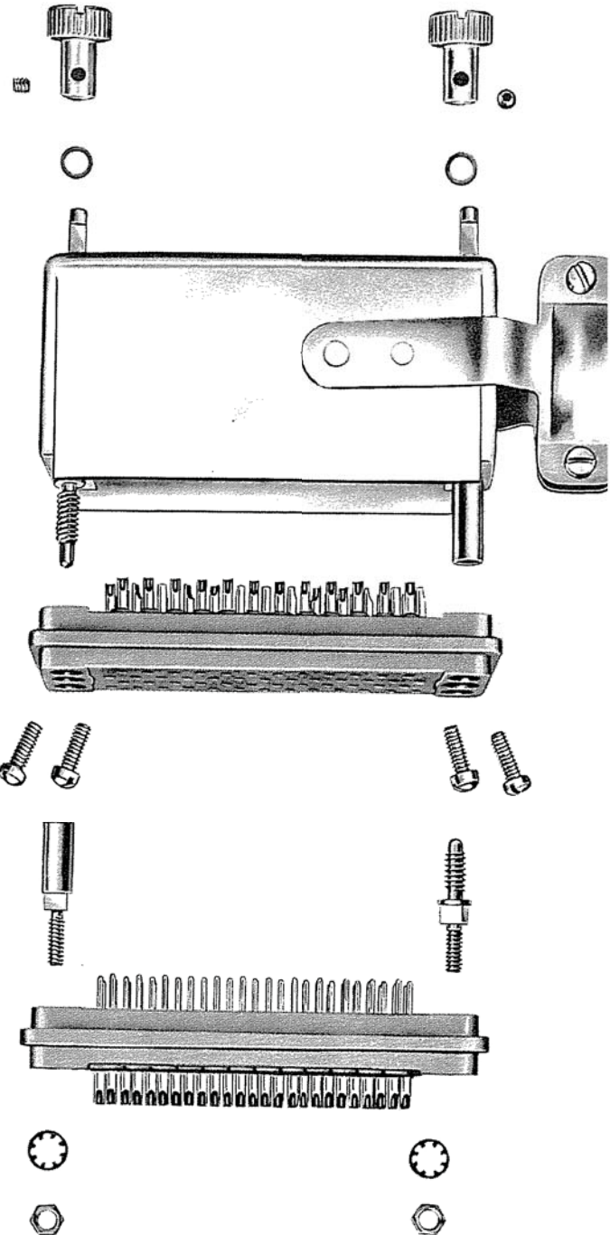
EXPLODED VIEW ACTUAL SIZE
