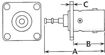
Figure 1 (Turret contact)
