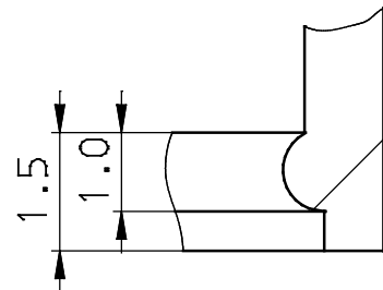
Einzelheit Z
